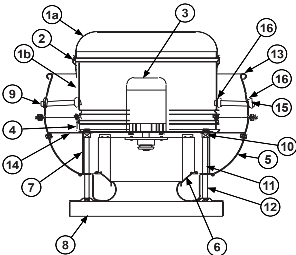
ACRU-D Sizes 101-195 C-Face
